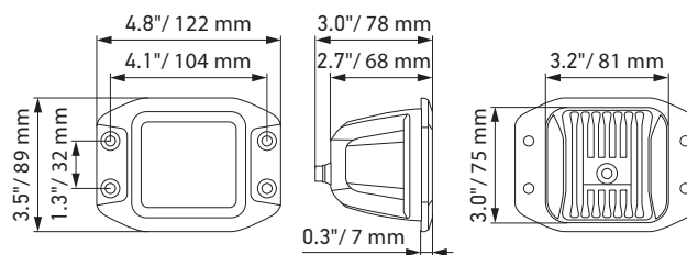
LED Cube 3,2" (wersja do montażu wpuszczanego)
