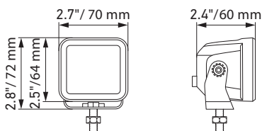
LED Cube 3,2" (wersja do montażu zewnętrznego)
