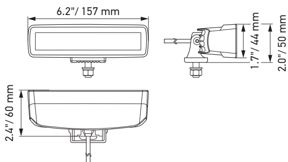
Wersja do montażu zewnętrznego
