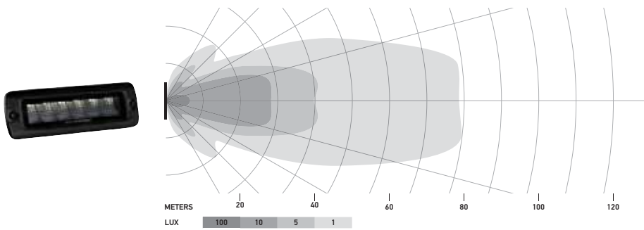
Black Magic Mini Lightbar 6,2" bliski zasięg, do zabudowy
