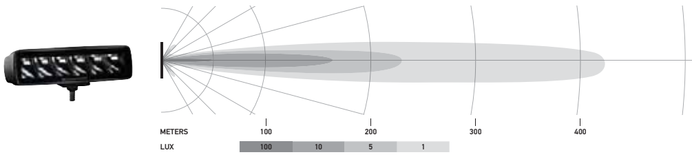
Black Magic Mini Lightbar 6,2" , daleki zasięg
