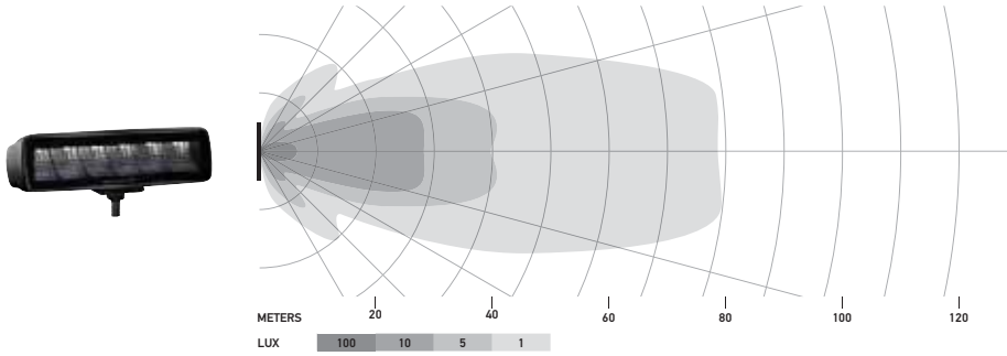
Black Magic Mini Lightbar 6,2" , bliski zasięg
