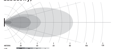
Zestaw LED Cube 3,2", bliski zasięg (do zabudowy)
