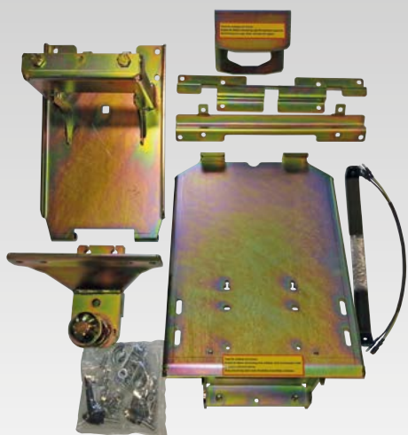
Uchwyt kombi do narzędzi oraz wzmocniony zaczep kulowy podwójny. Standardowy uchwyt do Grizzly 550/700 od 2014. Nr art. YFM77000
